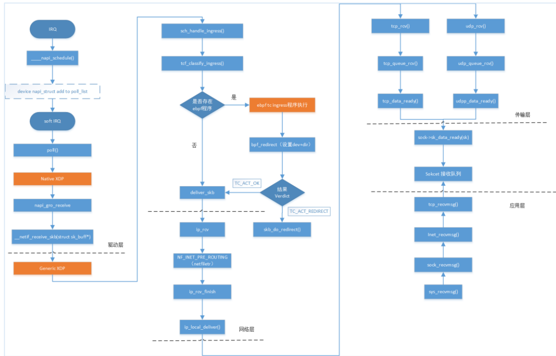
图 3-3-2 网络包收包流程示意图
