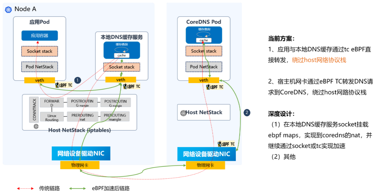
图 3-3-9 基于 TC eBPF 的流量转发路径示意图
