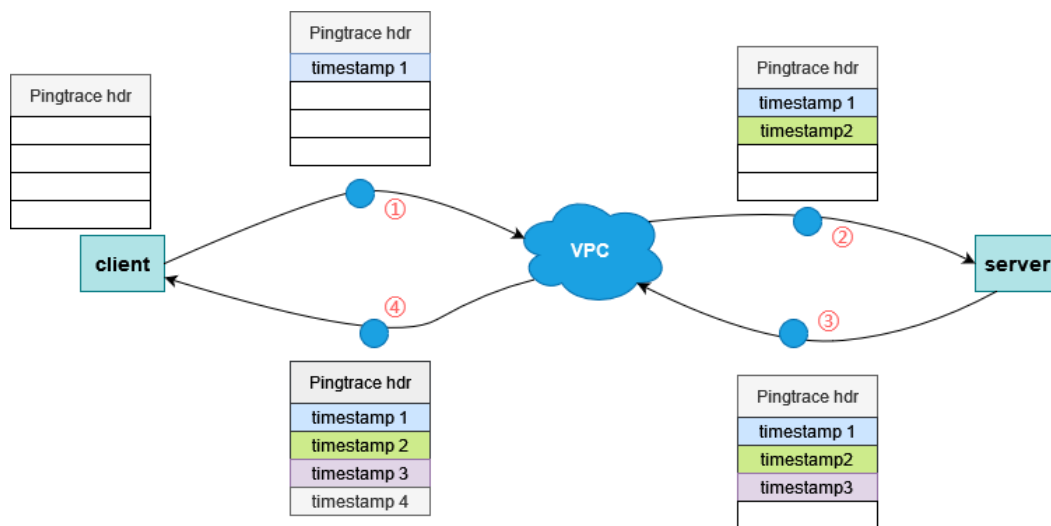
图 3-1-1 PingTrace 原理图
